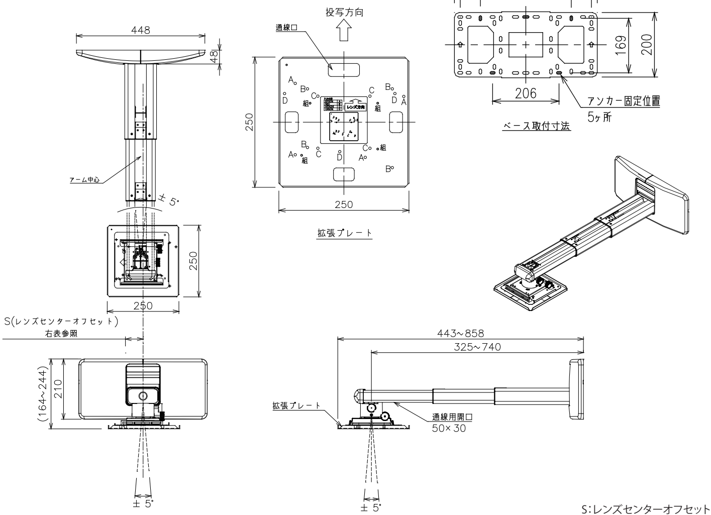
S: レンズセンターオフセット
