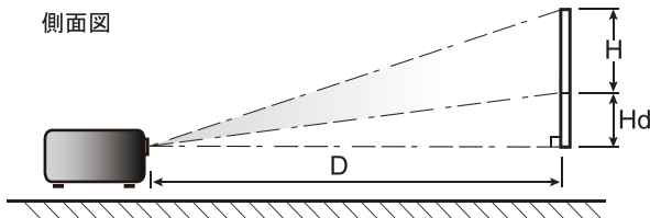
側面図
