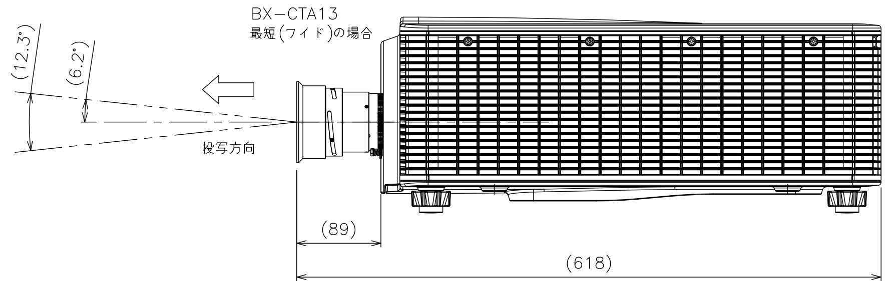
ZU1300装着時寸法(S=1:4)
