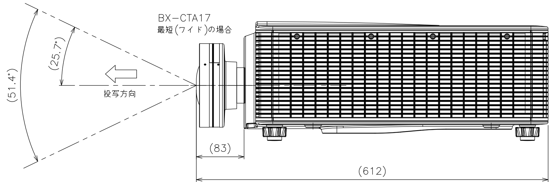
ZU1300装着時寸法(S=1:4)
