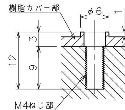
プロジェクター取付穴詳細図
